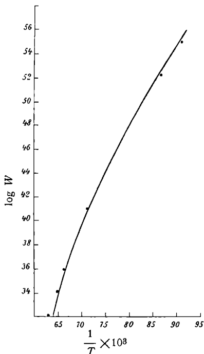
Fig. 5. Quarz I, dritte Erhitzung.
