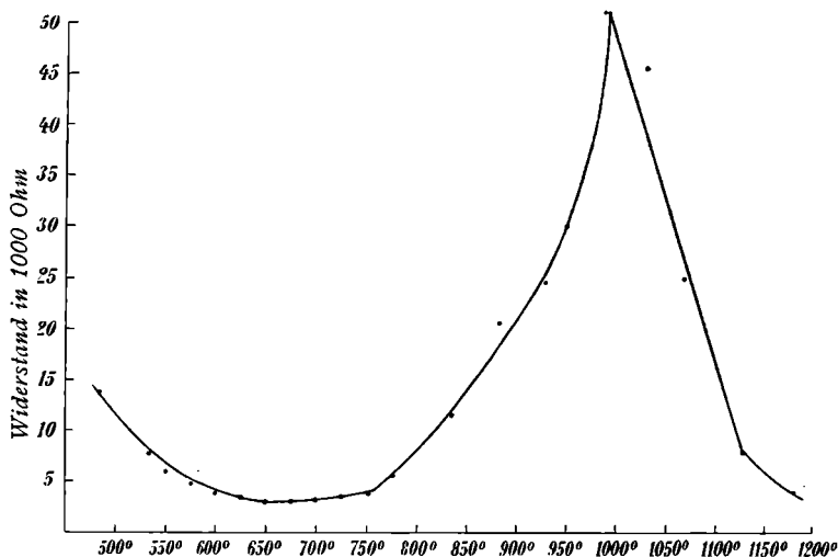
Fig. 3. Quarz I, zweite Erhitzung.
