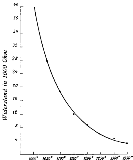
Fig. 16. Baryt.
