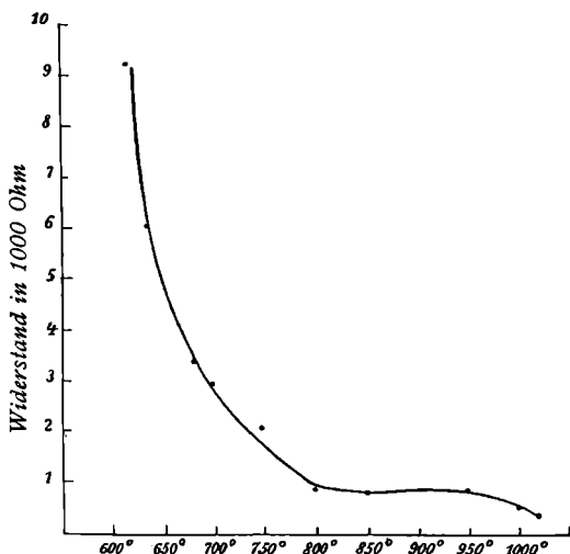
Fig. 13. Granat.
