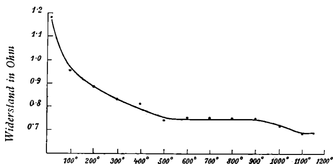
Fig. 11. Magneteisen.
