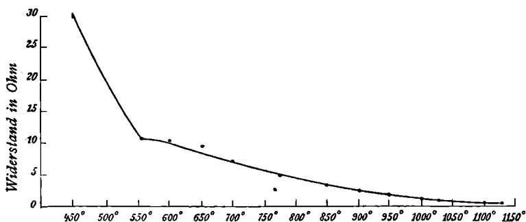
Fig. 18. Wolframit.
