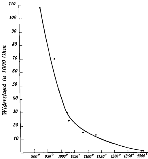
Fig. 4. Quarz I, dritte Erhitzung.
