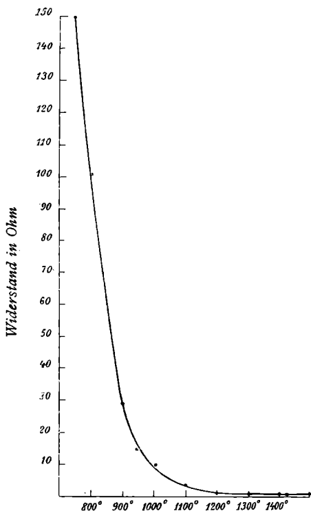
Fig. 1. Zinnstein.
