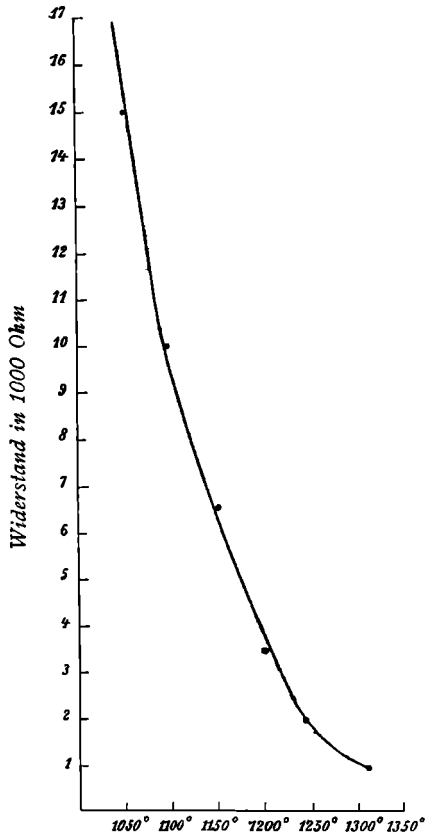
Fig. 7. Rauchquarz A.
