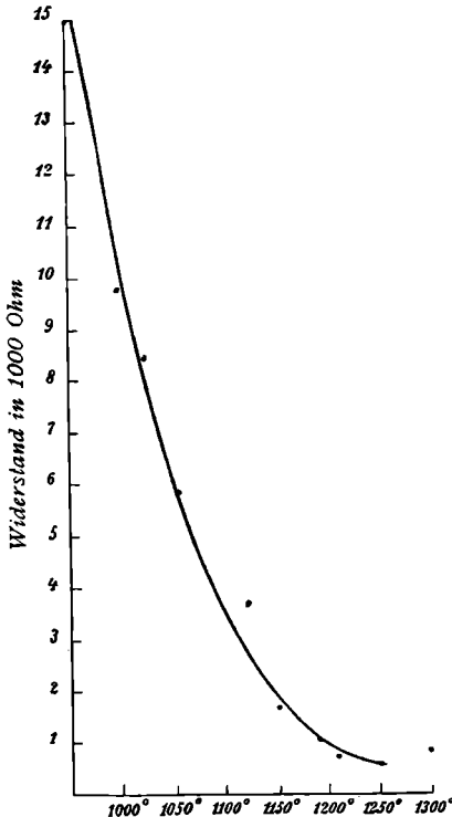
Fig. 8. Rauchquarz B.
