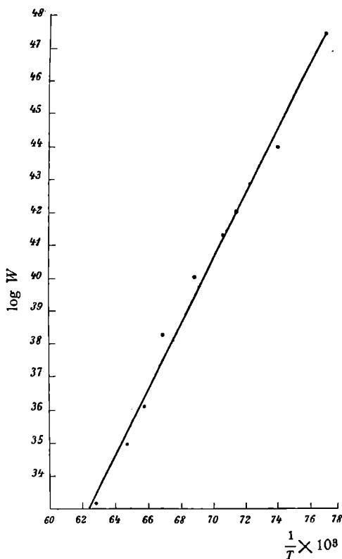
Fig. 15. Topas.
