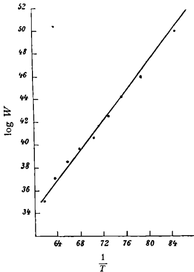
Fig. 17. Baryt.
