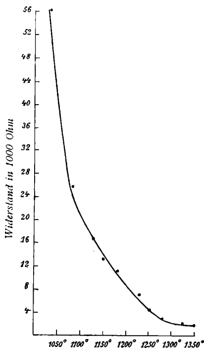
Fig. 14. Topas.
