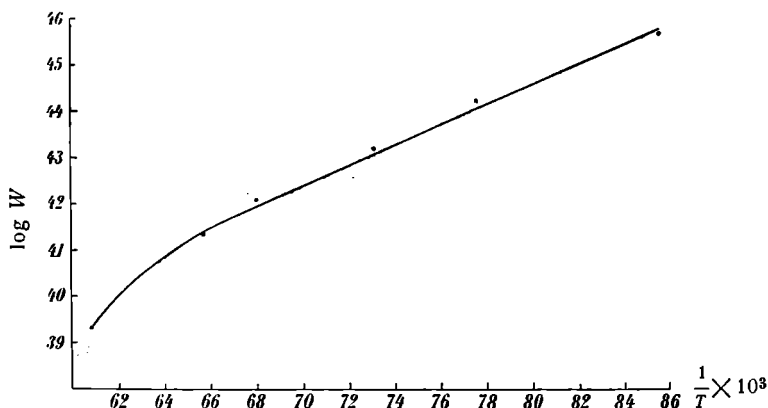
Fig. 12. Chrysoberyll.
