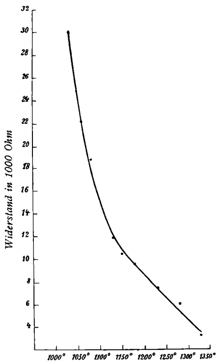
Fig. 9. Saphir.
